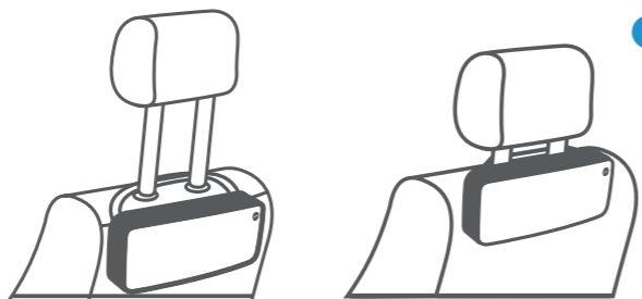
將主機綁帶套入頭枕支架後收緊綁帶
